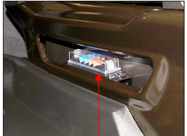
TAXI-Sicherungskasten
